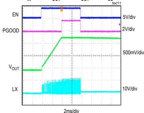
STARTUP/SOFTSTOP DISABLED
